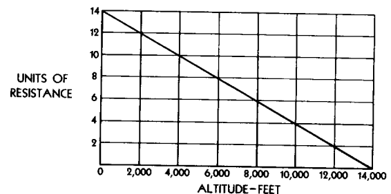
FIG. 11 ALTITUDE COMPENSATOR
